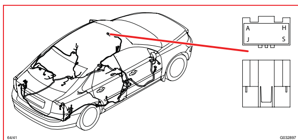
64/41 接頭
