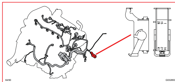
64/90 接頭
