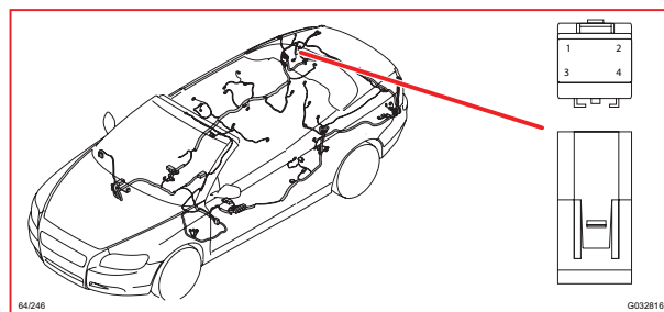
64/246 接頭
