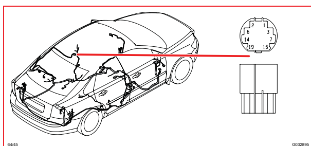
64/45 接頭
