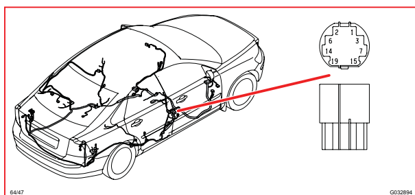
64/47 接頭
