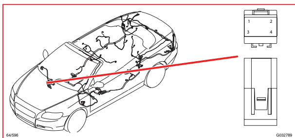
64/596 接頭
