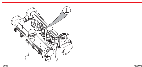
31/88 接地，引擎
