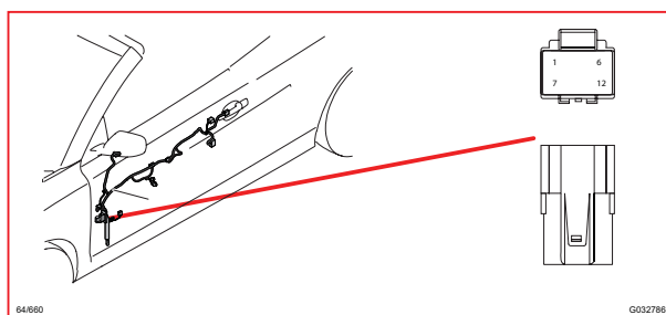
64/660 接頭
