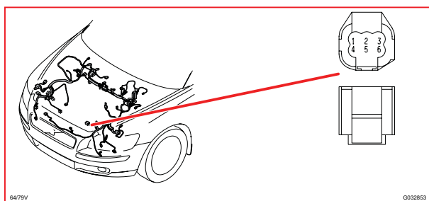
64/79V 接頭
