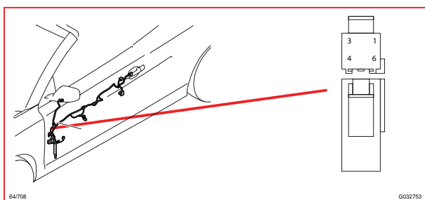
64/708 接頭
