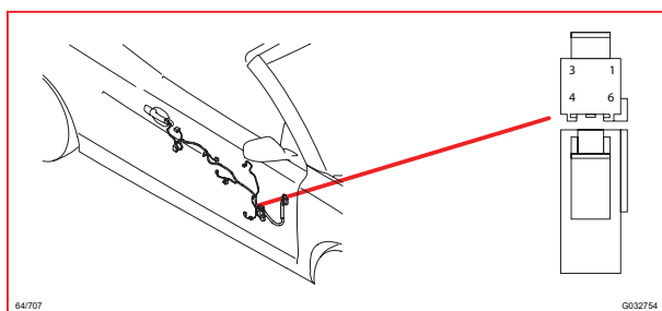
64/707 接頭
