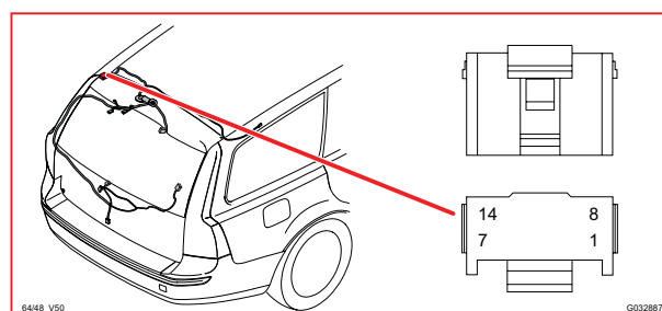
64/48 接頭，V50
