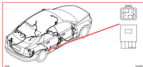
64/50 接頭
