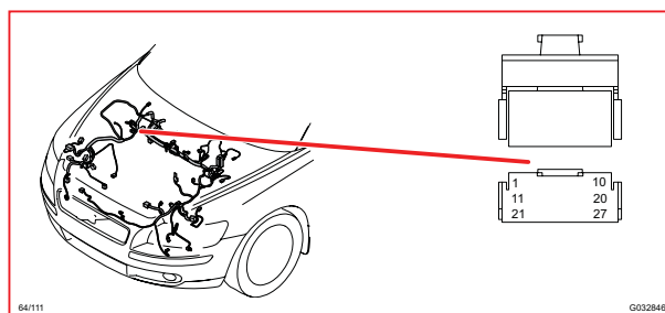
64/111 接頭
