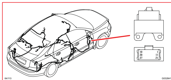
64/113 接頭
