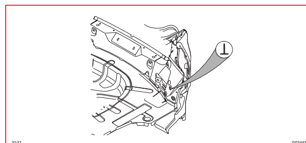
31/11 接地，左後側
