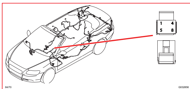
64/70 接頭
