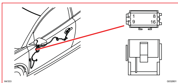
64/333 接頭
